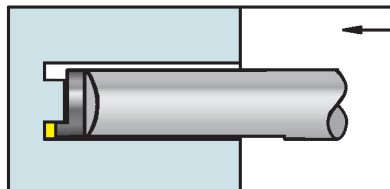
Axial grooving
