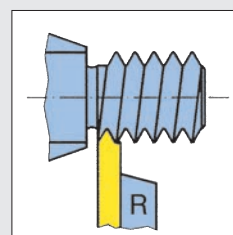
Gewinde Vollprofil
