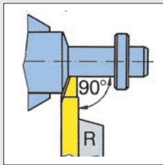
Einstecken Drehen
