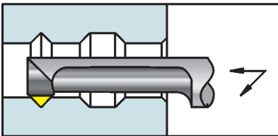
Fasen und Auskammern
