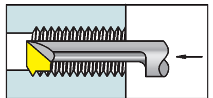
Gewindeschneiden
