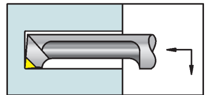
Drehstahl
