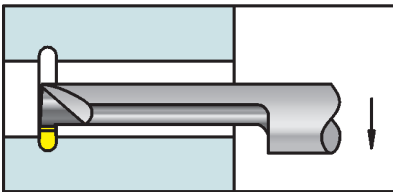
Stechdrehen Radius
