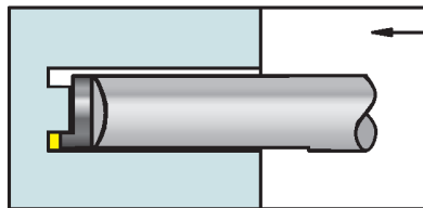
Axialstechen
