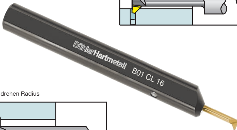
Rückwärtsdrehen
