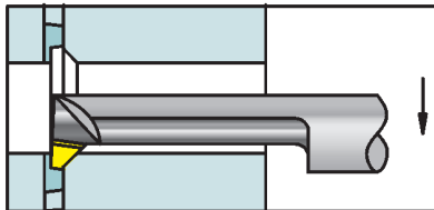
Vorstechen und Fasen
