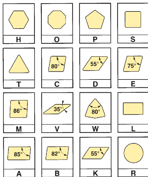
Plattenform
