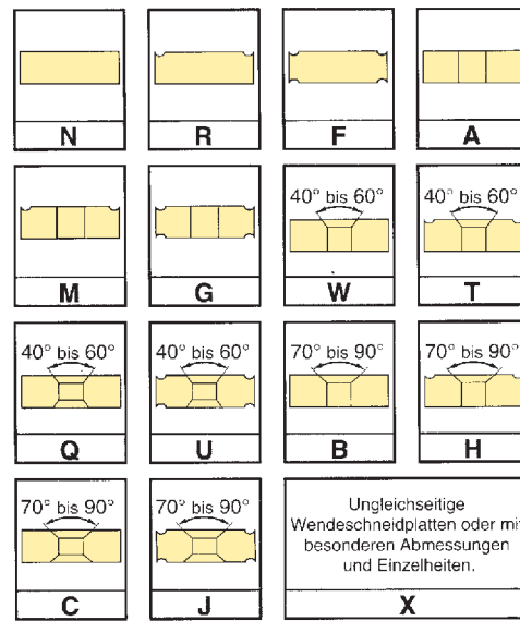
Befestigung - Schneidengeometrie
