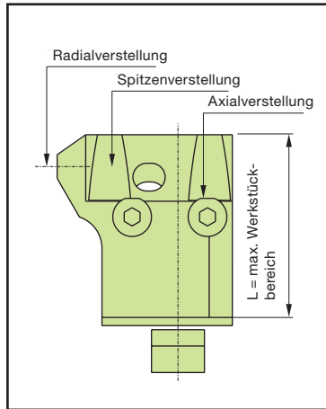
Aufsatzhalter X
