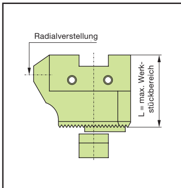
Aufsatzhalter A1
