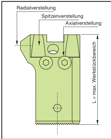
Aufsatzhalter A1
